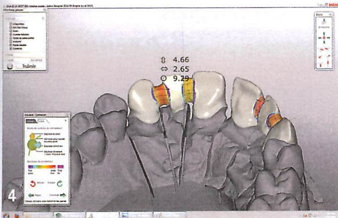
4. Diamètre requis des connexions des pontiques. Ici pour une connexion dans une armature zirconie environ 9 mm 2 .
